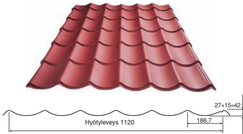
Terästiili 1120
