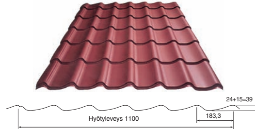
Teräsaalto 1100
